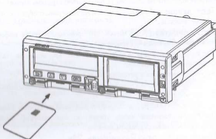
Рисунок 3 – Установка карты водителя в слот «Основной водитель»
