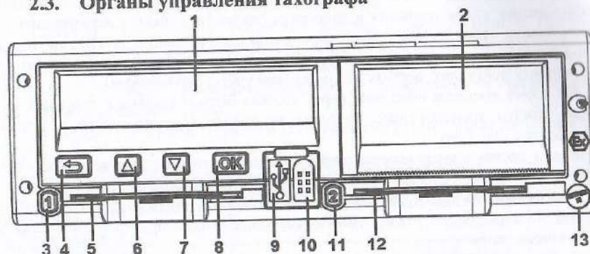
Рисунок 2 – Внешний вид передней панели тахографа.
